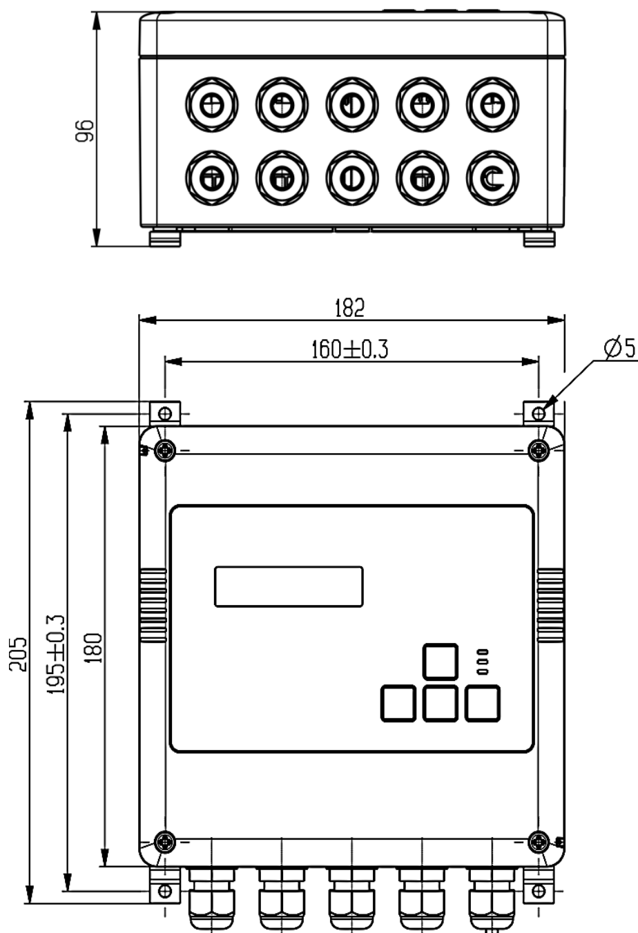
Рисунок Б.15 Габаритные и установочные размеры ПМ.03
