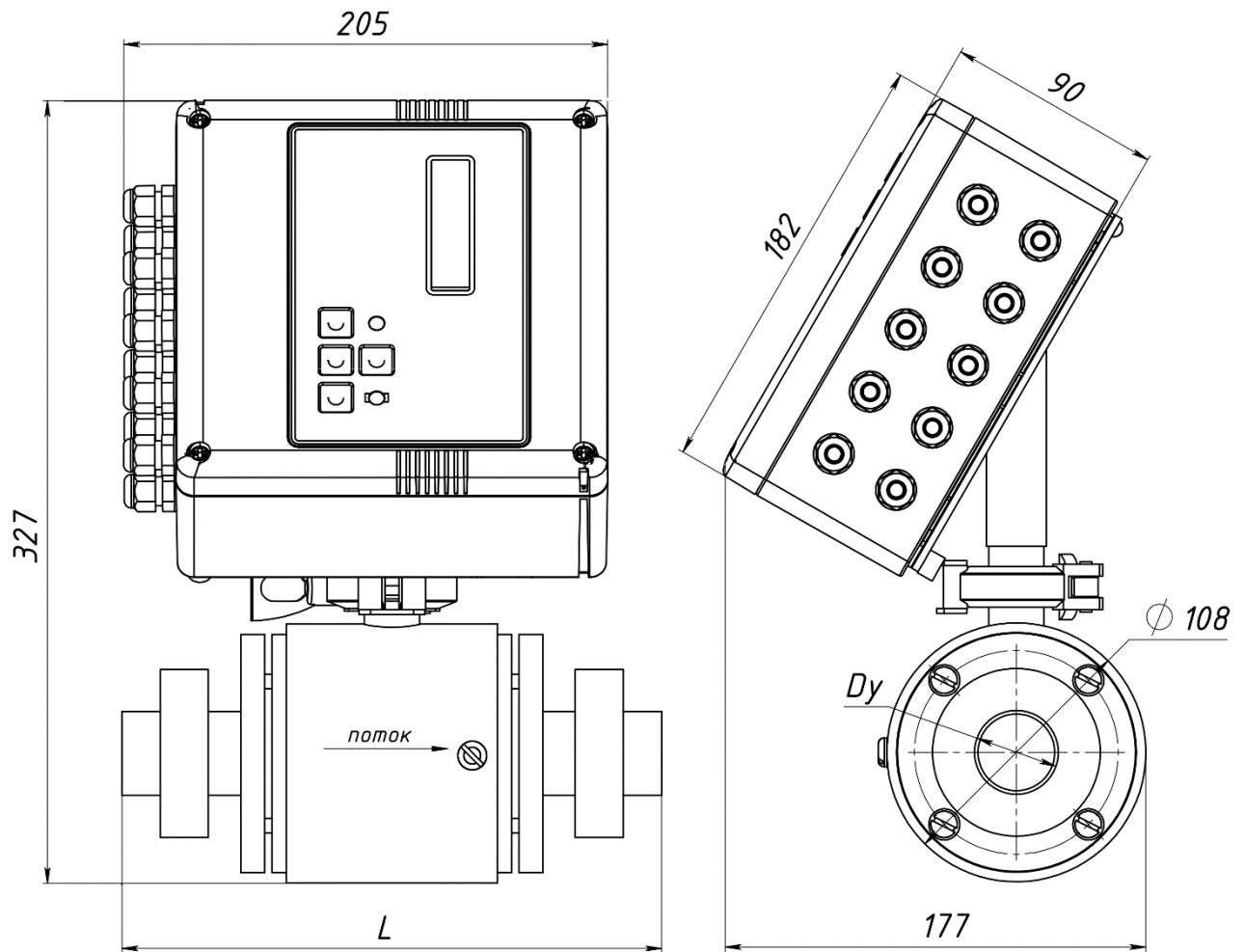
Рисунок Б.14 Расходомер совмещенного исполнения при установке на вертикальном участке трубопровода (по заказу любой тип ППР и вид соединения)
