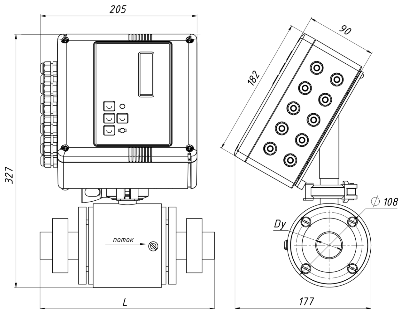
Рисунок Б.13 Расходомер совмещенного исполнения при установке на вертикальном участке трубопровода (по заказу любой тип ППР и вид соединения)
