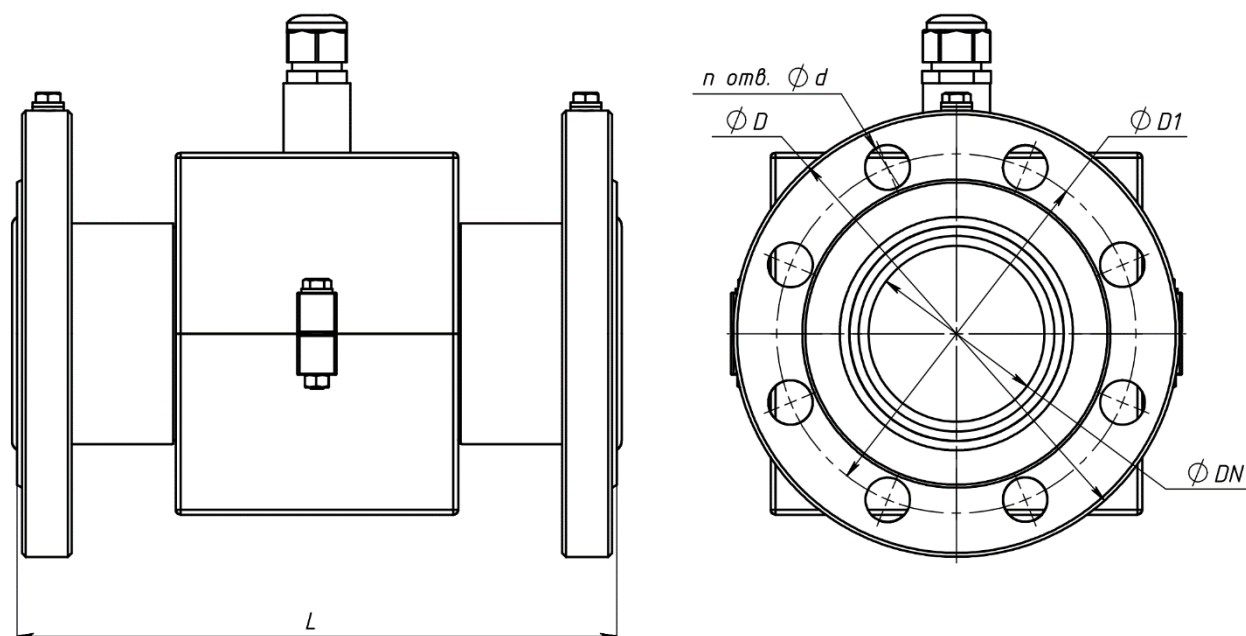
Рисунок Б.5 Габаритные и установочные размеры ПП
