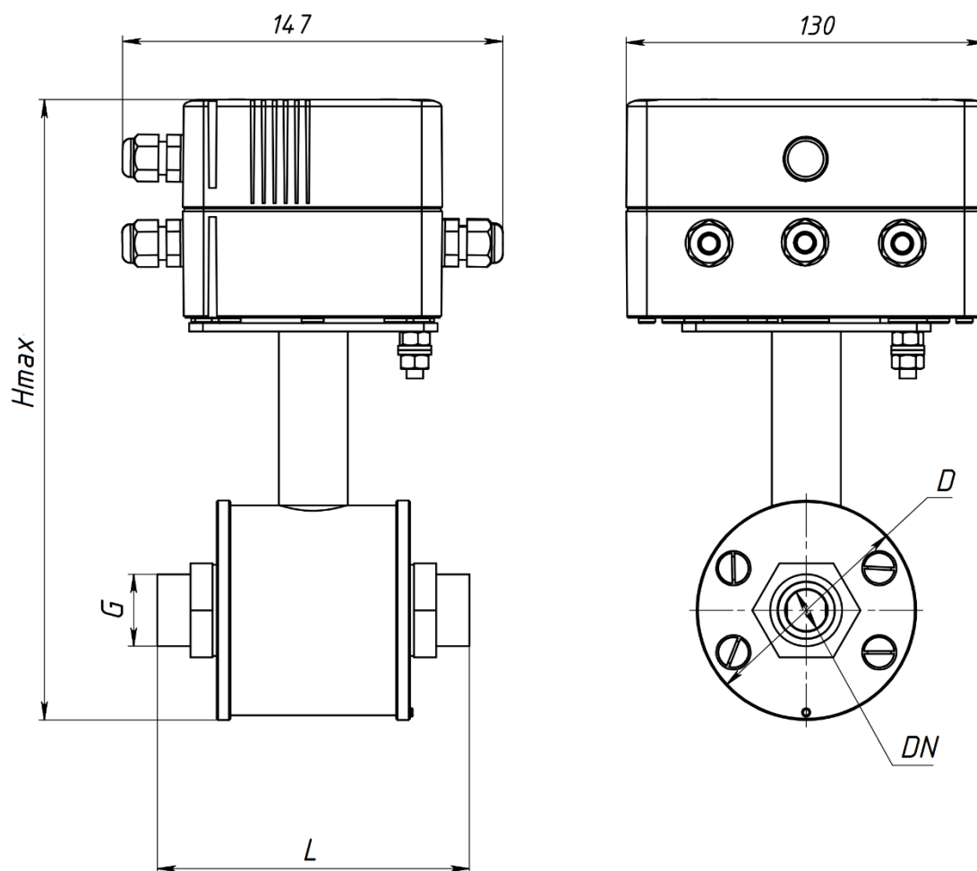
Рисунок Б.3 Габаритные и установочные размеры расходомеров РСМ-05.05(ТЭСМАРТ-П), РСМ-05.05(ТЭСМАРТ-ПА) с ПМ.07.02 и ПРПН/Р
